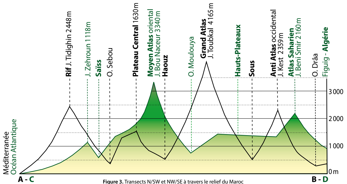
Figure 3. Transects N/SW et NW/SE à travers le relief du Maroc
