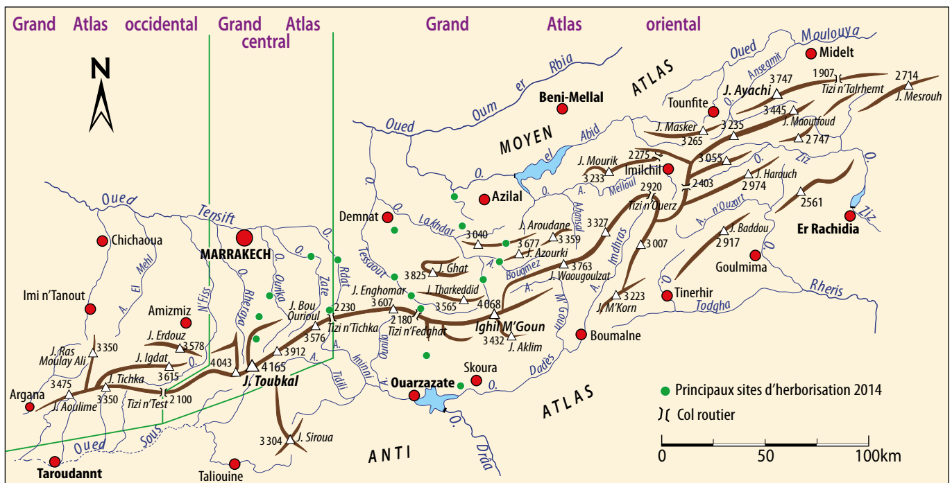
Figure 4. Carte schématique du Grand Atlas, d'après QUEZEL (1957), modifiée.
