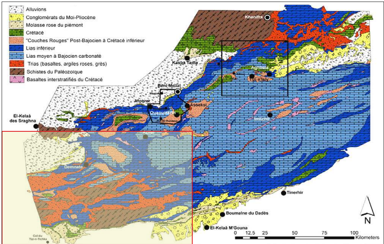
Figure 6. Carte géologique simplifiée du Grand Atlas central, d'après PROUST et al. (1977) et HOLLARD et al. (1985).
