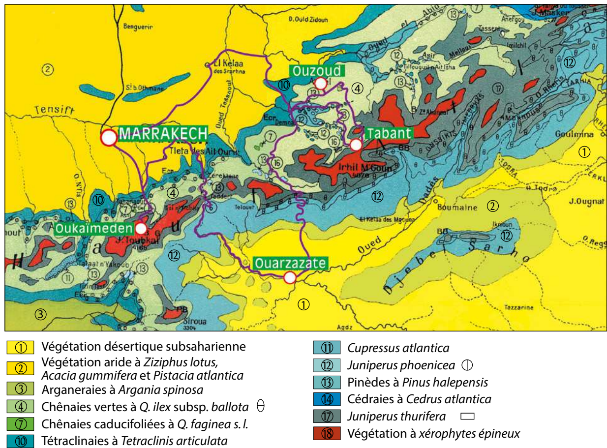
Figure 10. Extrait de la carte phytogéographique du SW du Maroc d'après L. EMBERGER (1939) et itinéraires de la session, ○ localité-étape.
